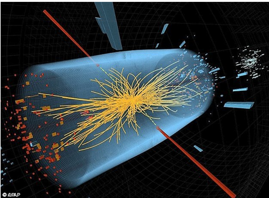
Afbeelding 4. Simulatie van een botsing tussen twee quantumdeeltjes.
